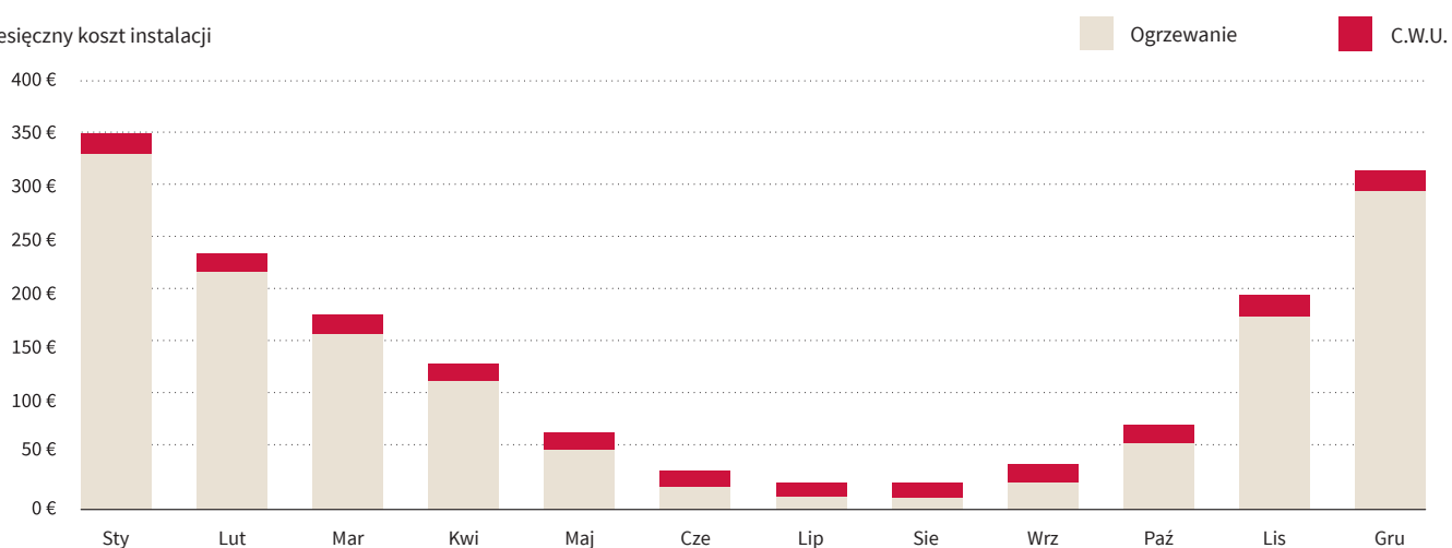
Porównanie kosztów zużycia energii przez pompę Yutaki z tradycyjnymi instalacjami grzewczymi
